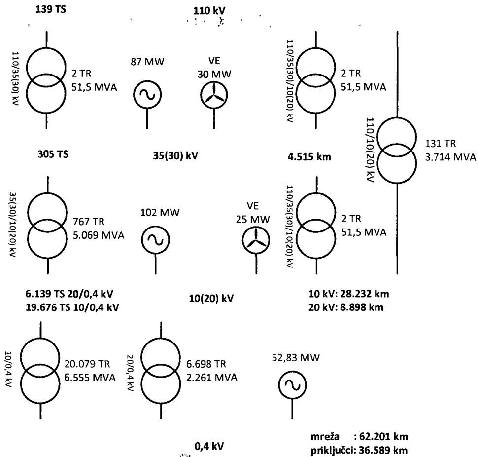
Slika 4.2.2. Osnovni podaci o distribucijskom sustavu na dan 31. prosinca 2017. godine
