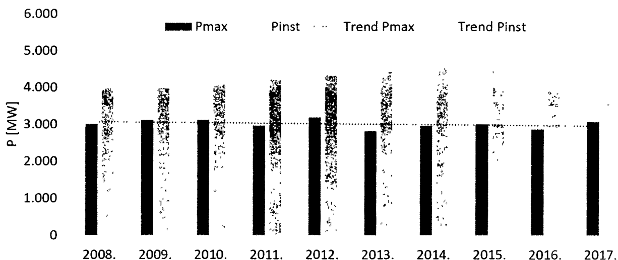
Slika 4.5.3. Prikaz maksimalnog opterećenja hrvatskog elektroenergetskog sustava ( P_{max} ) i snage elektrana na području Republike Hrvatske ( P_{inst} ) od 2008. do 2017. godine
