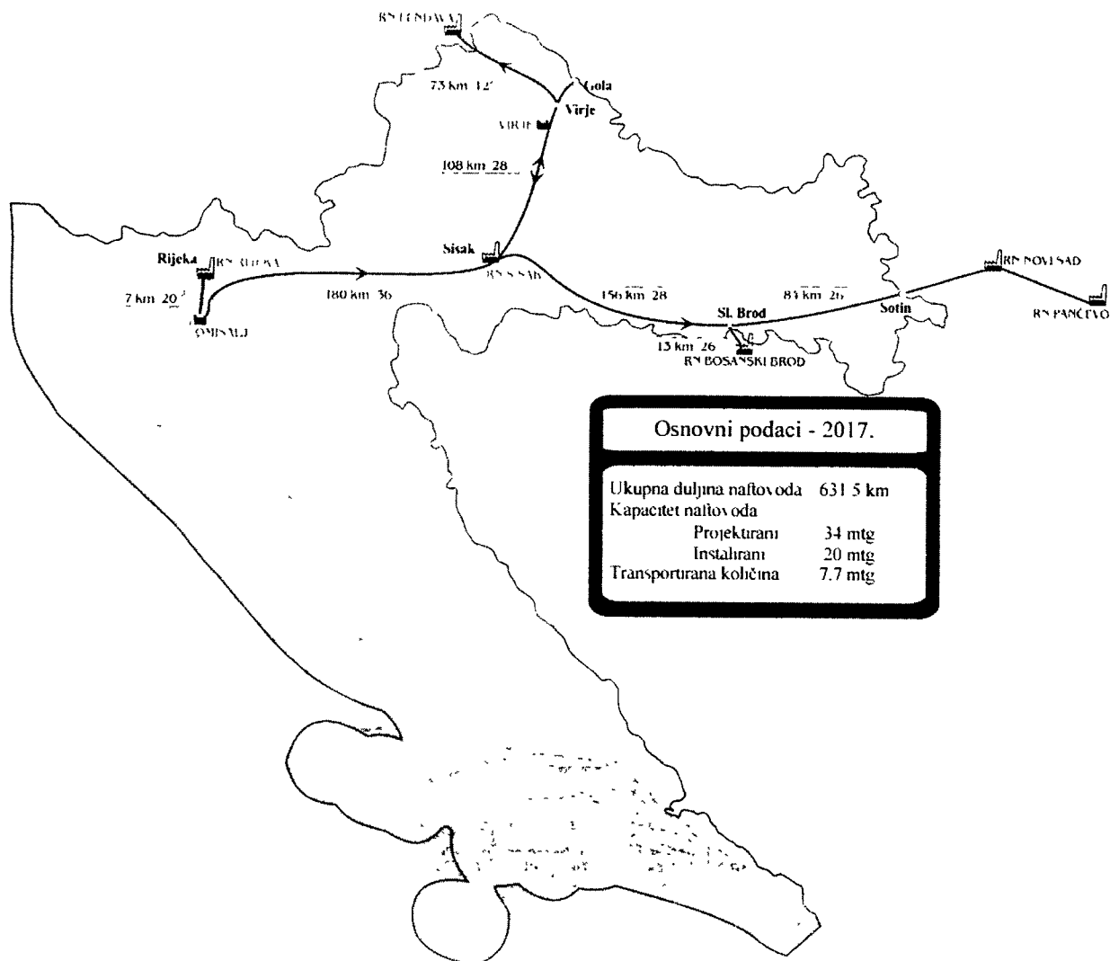
Slika 6.2.1. Naftovodni sustav JANAFT-a d.d.
