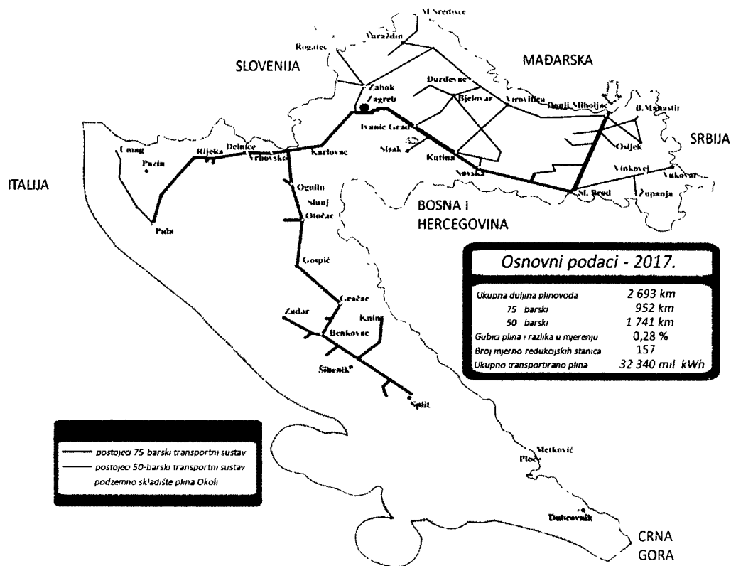
Slika 5.2.1. Plinski transportni sustav Republike Hrvatske
