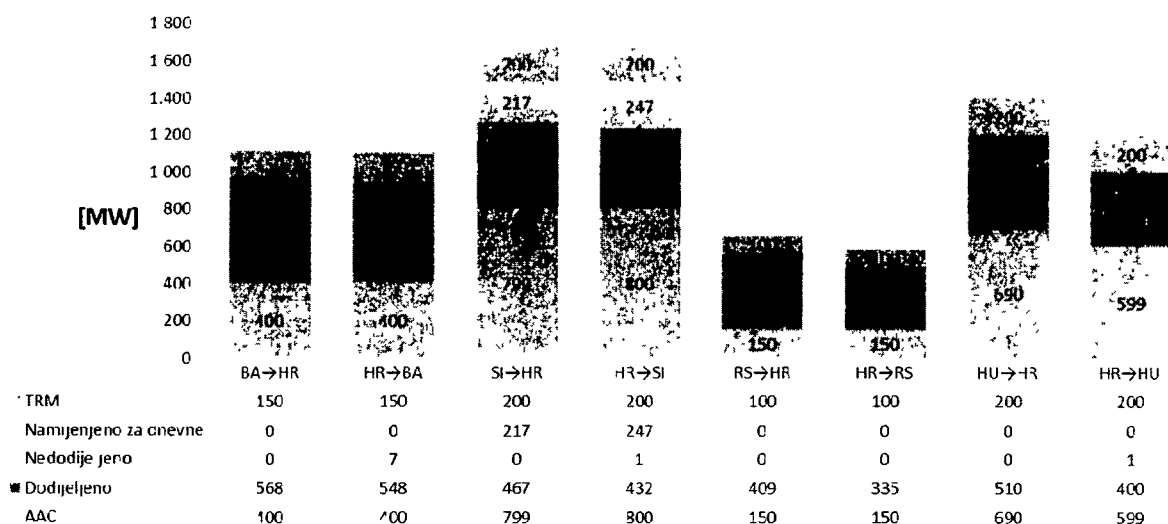
Slika 4.3.4. Prosječne mjesečne vrijednosti prekozonskih kapaciteta po granicama u 2017. godini
