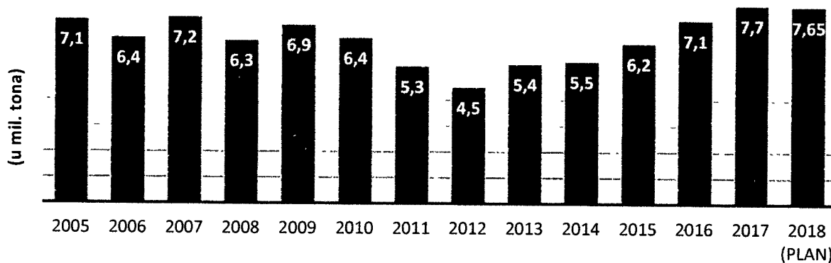
Slika 6.2.2. Naftovodni sustav JANAFT-a – transportirane količine [mil.t]
