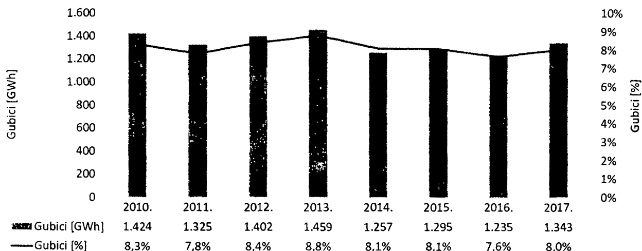
Slika 4.2.5. prikazuje iznose i postotke gubitaka u distribucijskoj mreži u razdoblju od 2010. do 2017. godine.
