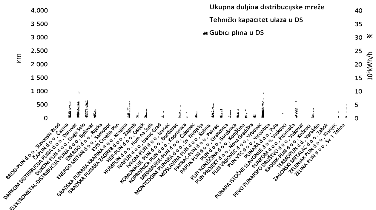
Slika 5.2.7. Usporedba duljine distribucijskih sustava, ukupnog tehničkog kapaciteta ulaza u distribucijske sustave i gubitaka plina po operatorima distribucijskog sustava u Republici Hrvatskoj u 2017. godini
